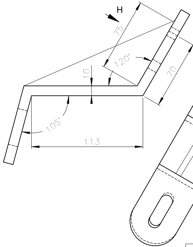
VISTA H
