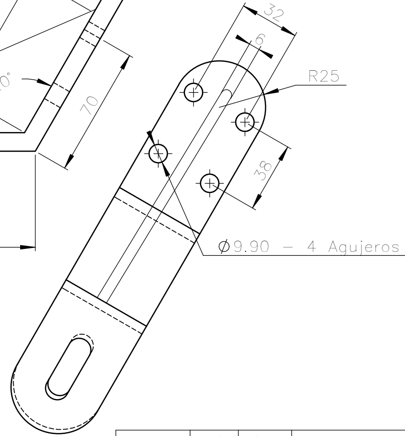
VISTA H
