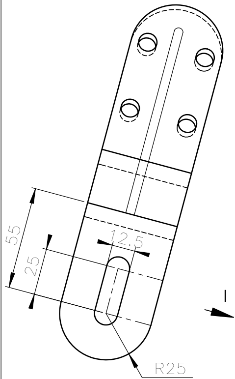
VISTA I
